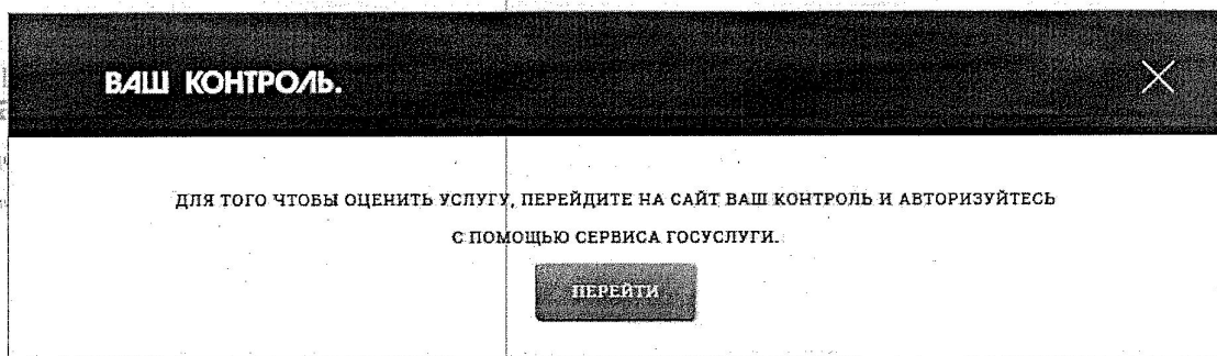
Рисунок 10. Окно виджета
