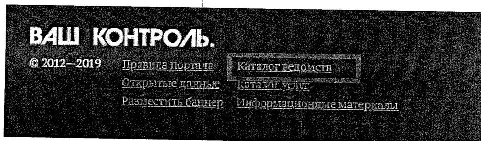
Рисунок 2. Каталог ведомств
