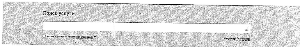
Рисунок 1. Поиск услуг
